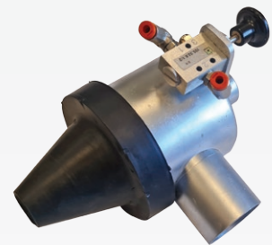
Głowica komplet Mobile
